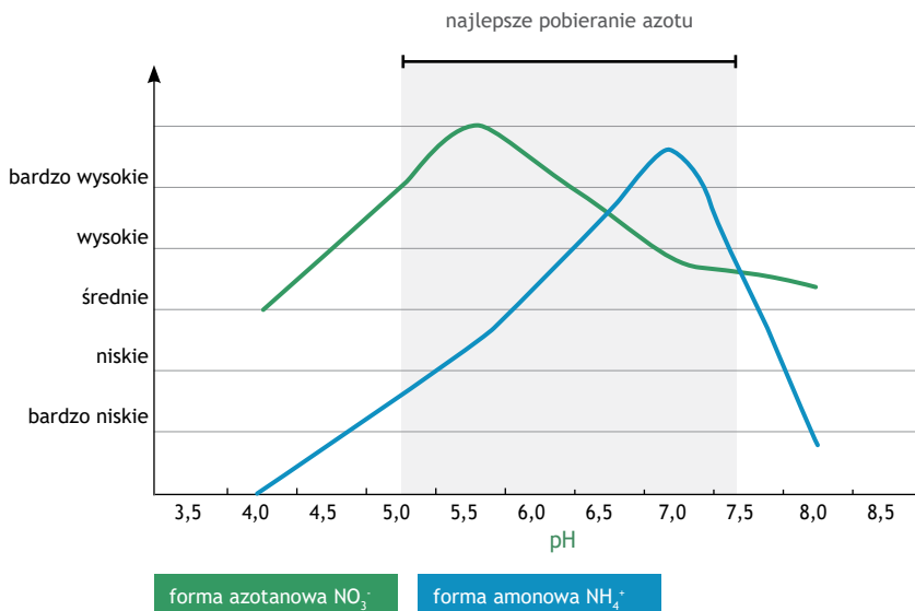
Rys. 5. Symulacja szybkości pobierania form azotu (N) w zależności od pH.
