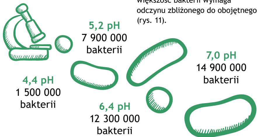
Rys. 10. Wpływ odczynu gleby na liczbę bakterii glebowych. jednostka szt./1g gleby
